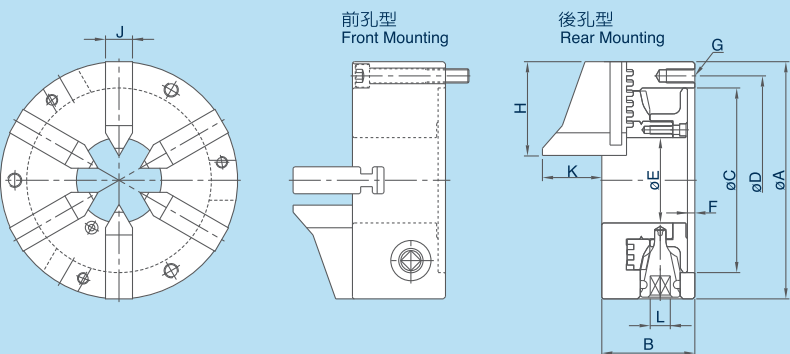
尺寸圖 » Dimensions
