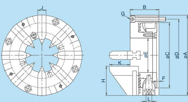
尺寸圖 » Dimensions
