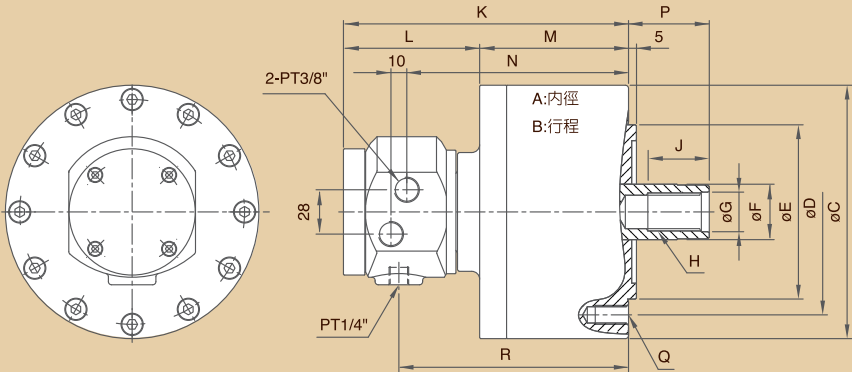
尺寸圖 » Dimensions
