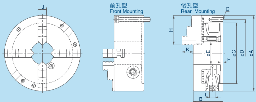
尺寸圖 » Dimensions
