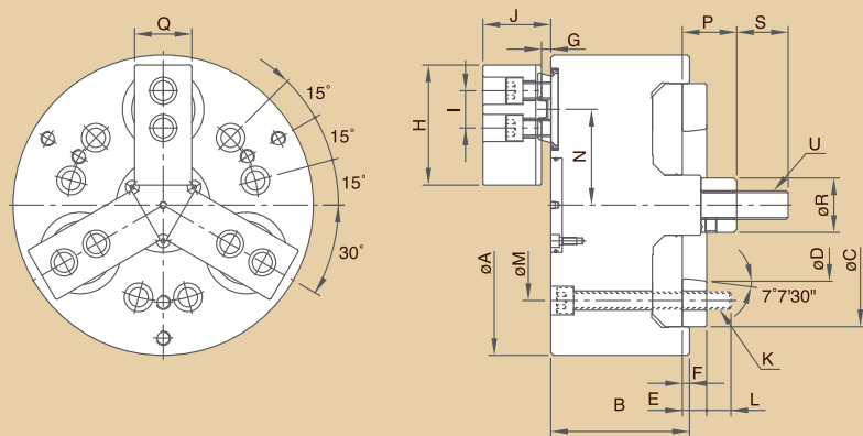
尺寸圖 » Dimensions
