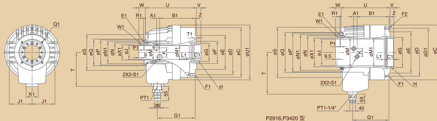
尺寸圖 » Dimensions
