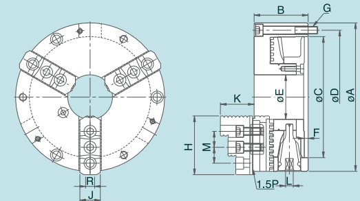
尺寸圖 » Dimensions
