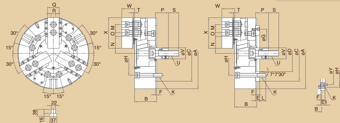
尺寸圖 » Dimensions
