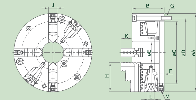
尺寸圖 » Dimensions
