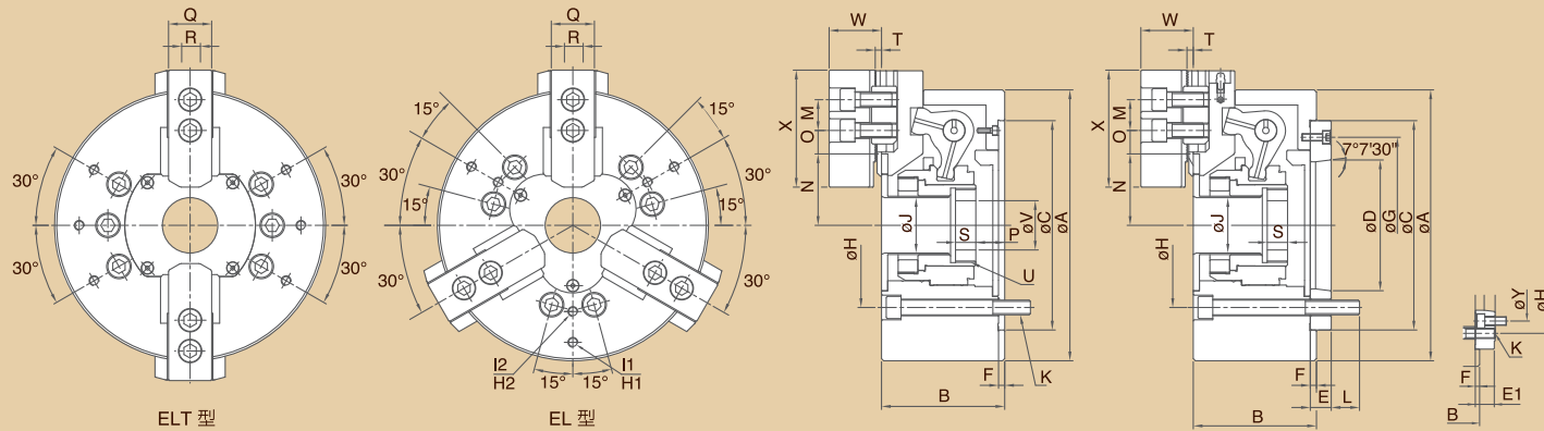
尺寸圖 » Dimensions
