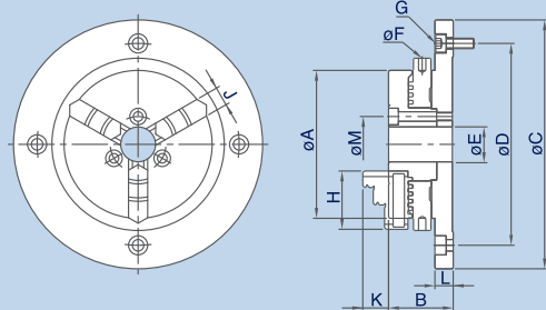
尺寸圖 » Dimensions
