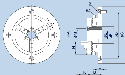
尺寸圖 » Dimensions
