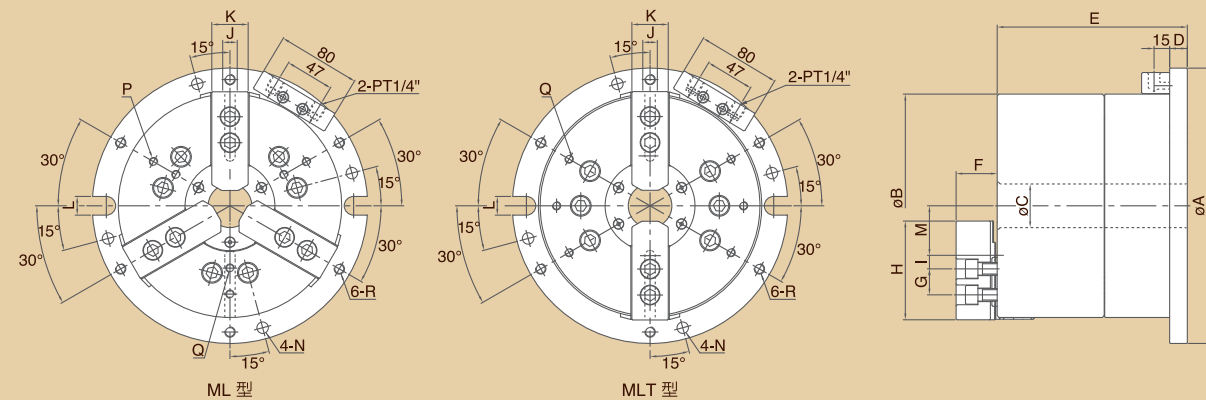
尺寸圖 » Dimensions
