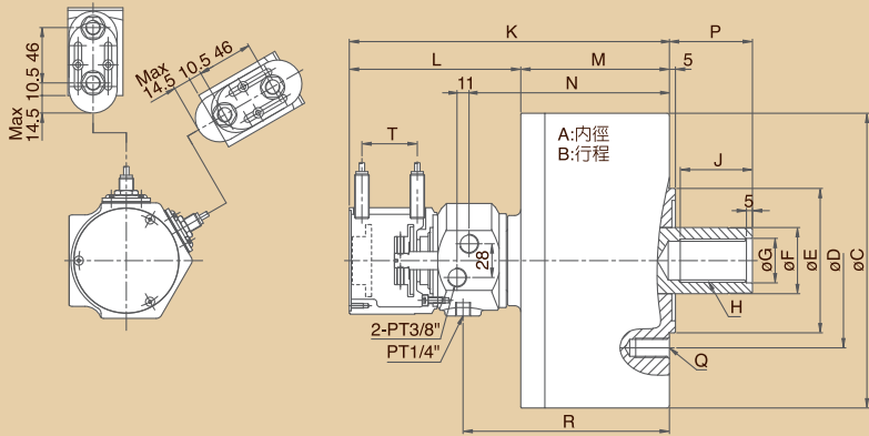
尺寸圖 » Dimensions
