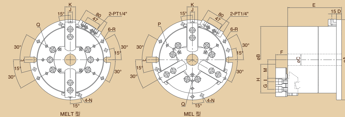
尺寸圖 » Dimensions
