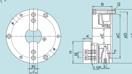
尺寸圖 » Dimensions
