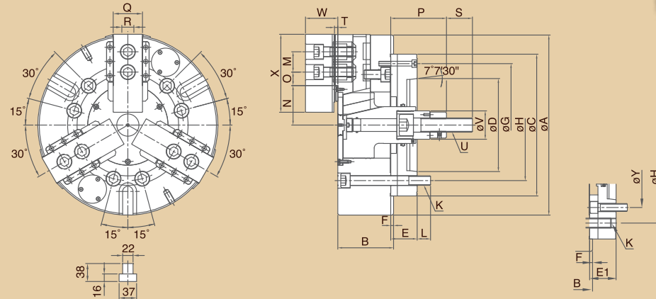
尺寸圖 » Dimensions
