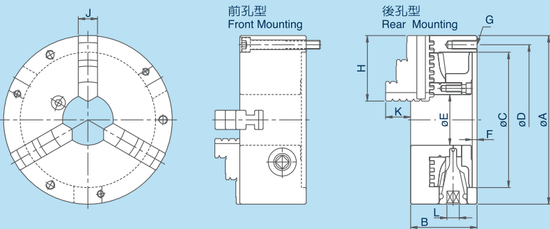
尺寸圖 » Dimensions
