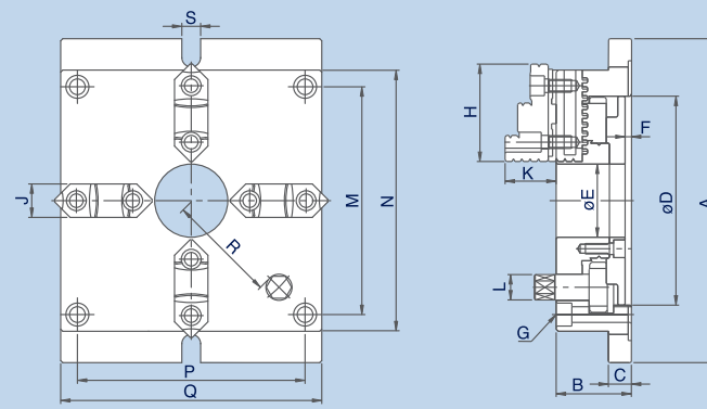
尺寸圖 » Dimensions
