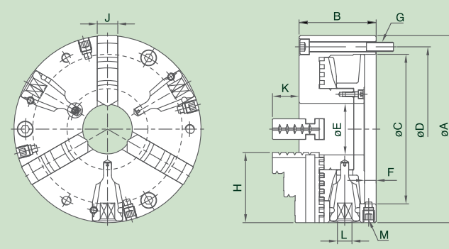
尺寸圖 » Dimensions
