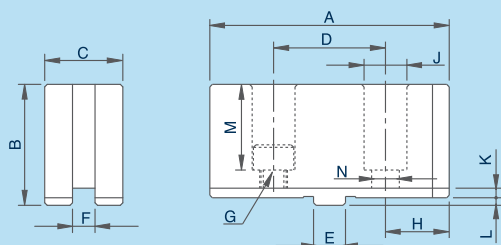
尺寸圖 » Dimensions
