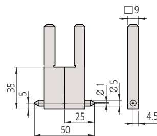
Внутренние точечные губки
