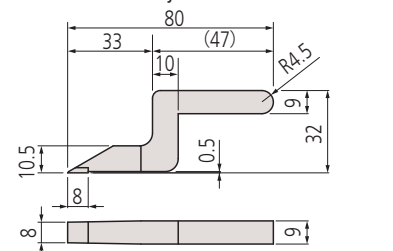
Разметочная ножка для штангенрейсмасов
