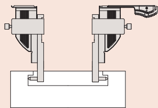
внутренний размер паза
